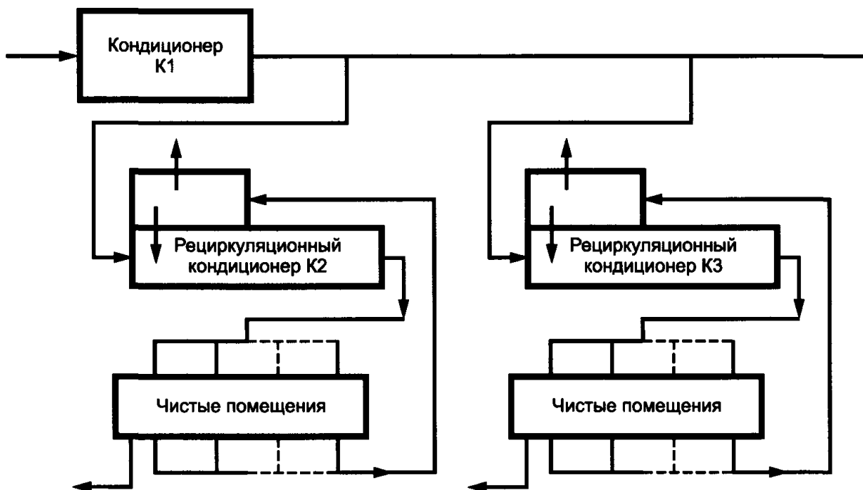
Рисунок А.4 - Двухуровневая система вентиляции и кондиционирования
