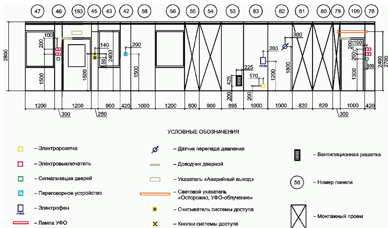
Рисунок 1 - Развертка стены чистого помещения
